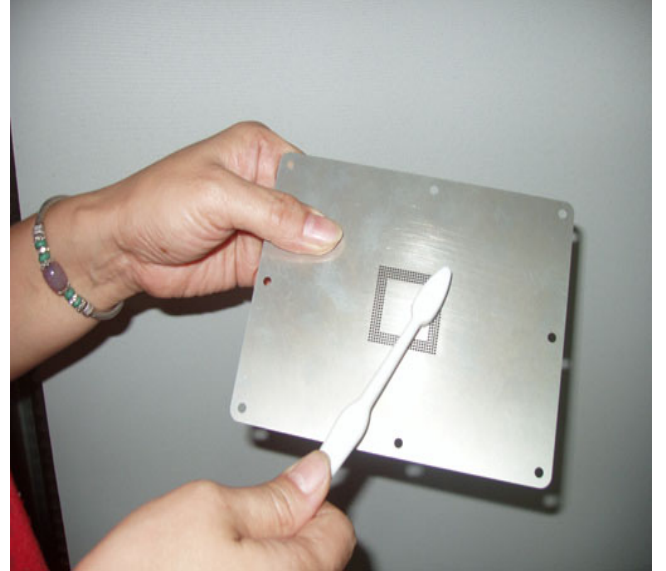
以牙刷沾溶劑清潔鋼板
