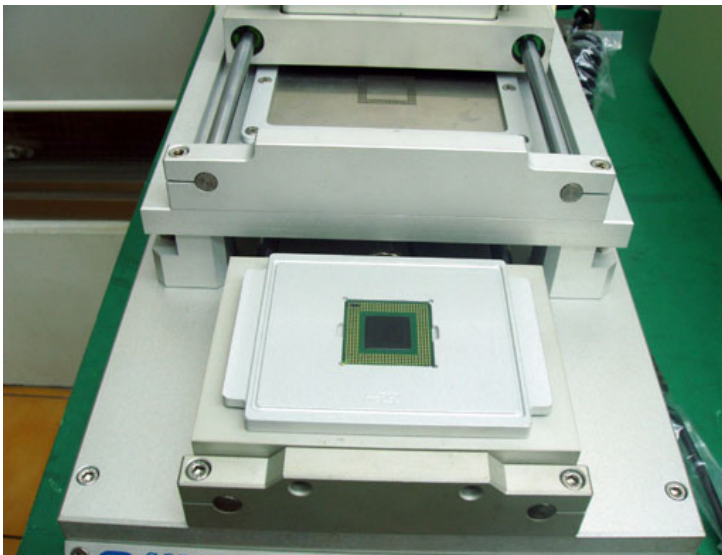
BGA 模具座槽與錫球模具座
