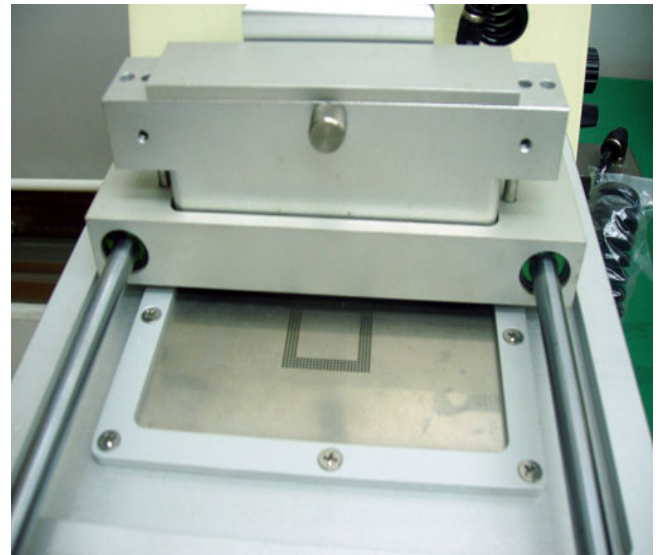
錫球模具與植球毛刷座
