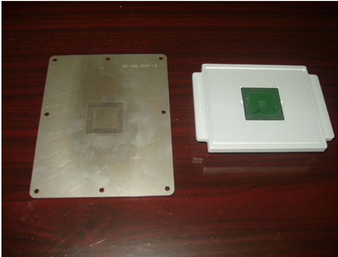
錫球模具與 BGA 模具
