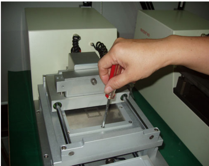
換新規格放回壓片上緊螺絲
