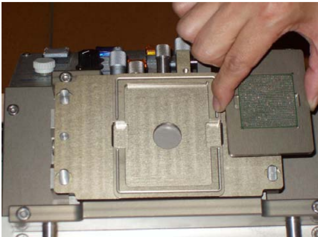
子內模具與主模具槽組合
