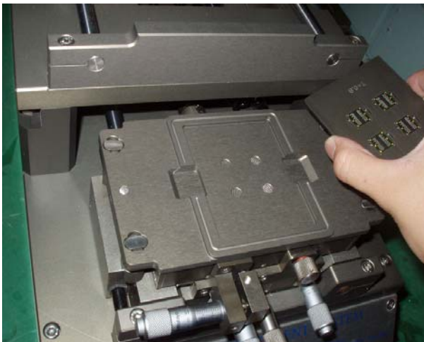
子內模具與主模具槽組合
